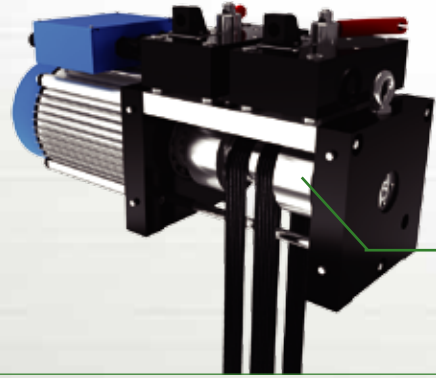
WRAP ANGLE 180° 包角180度
